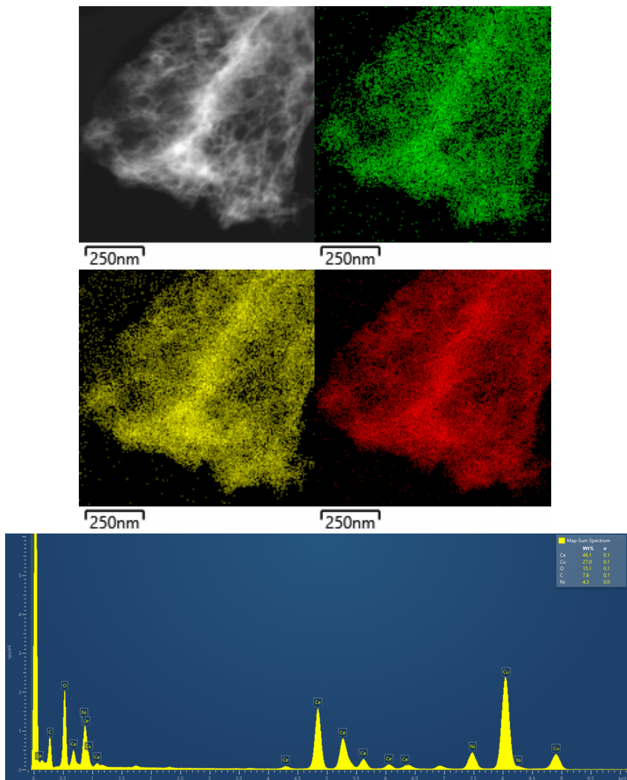
Figura 4.13: Mapeamento elemental e espectro de EDX para a amostra 10 % Ni@CeO 2 . Elementos: Ni (verde), O (amarelo) e Ce (vermelho).
