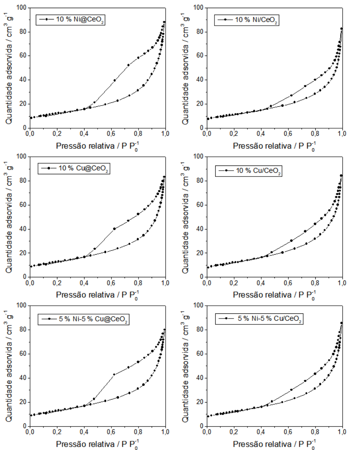
Figura 4.4: Isotermas de adsorção e dessorção de N 2 dos catalisadores.
