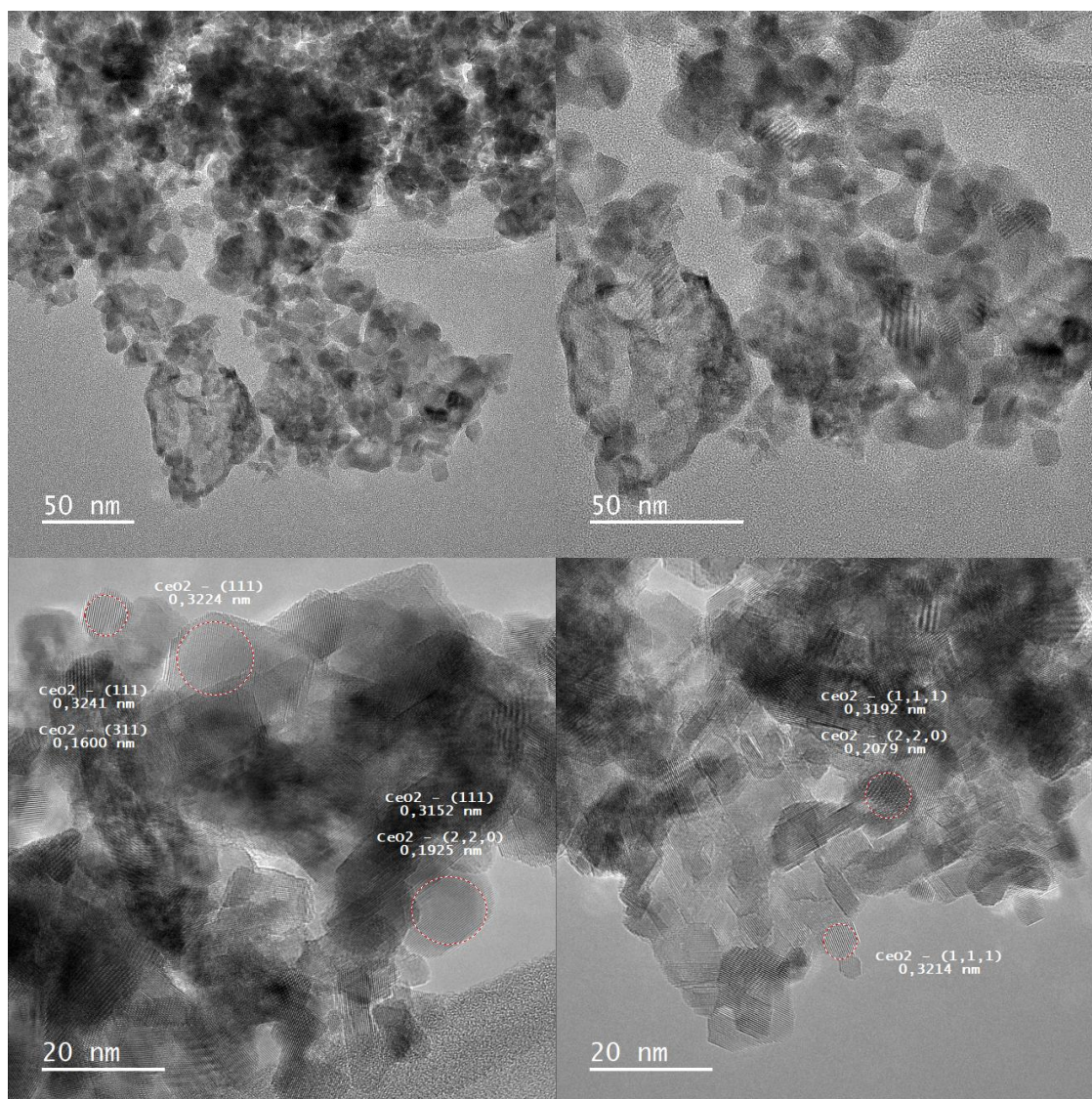
Figura 4.11: Imagens de MET para a amostra de \text{CeO}_2 .
