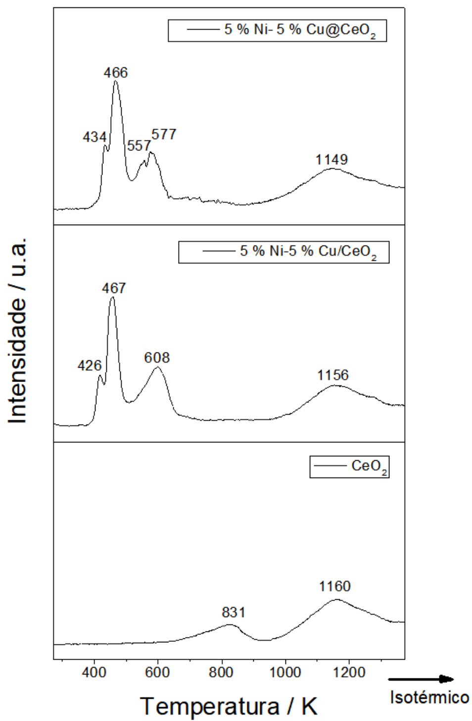
Figura 4.8: Perfis de RTP – 10 % H 2 /He para os catalisadores de Ni-Cu.
