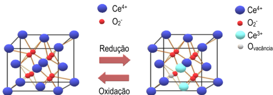
Figura 2.13: Capacidade redox do \text{CeO}_2 e sua influência na criação de vacâncias de oxigênio. Adaptado de: (MALAVASI et al. , 2010).
