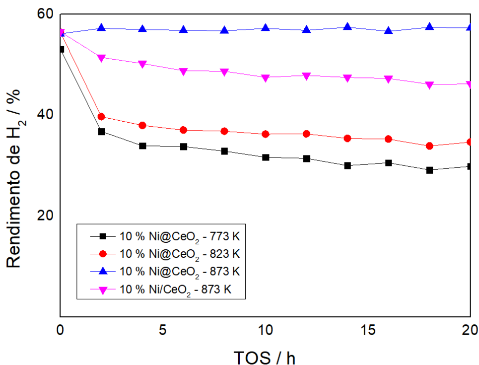
Figura 4.20: Rendimento de H_2 dos catalisadores embutidos e suportados de Ni. As reações foram conduzidas em 1 bar, a 773 K, 823 K e 873 K por 20 h com um GHSV de 492.000 \text{ mL} \cdot \text{h}^{-1} \cdot \text{gcat}^{-1} .
