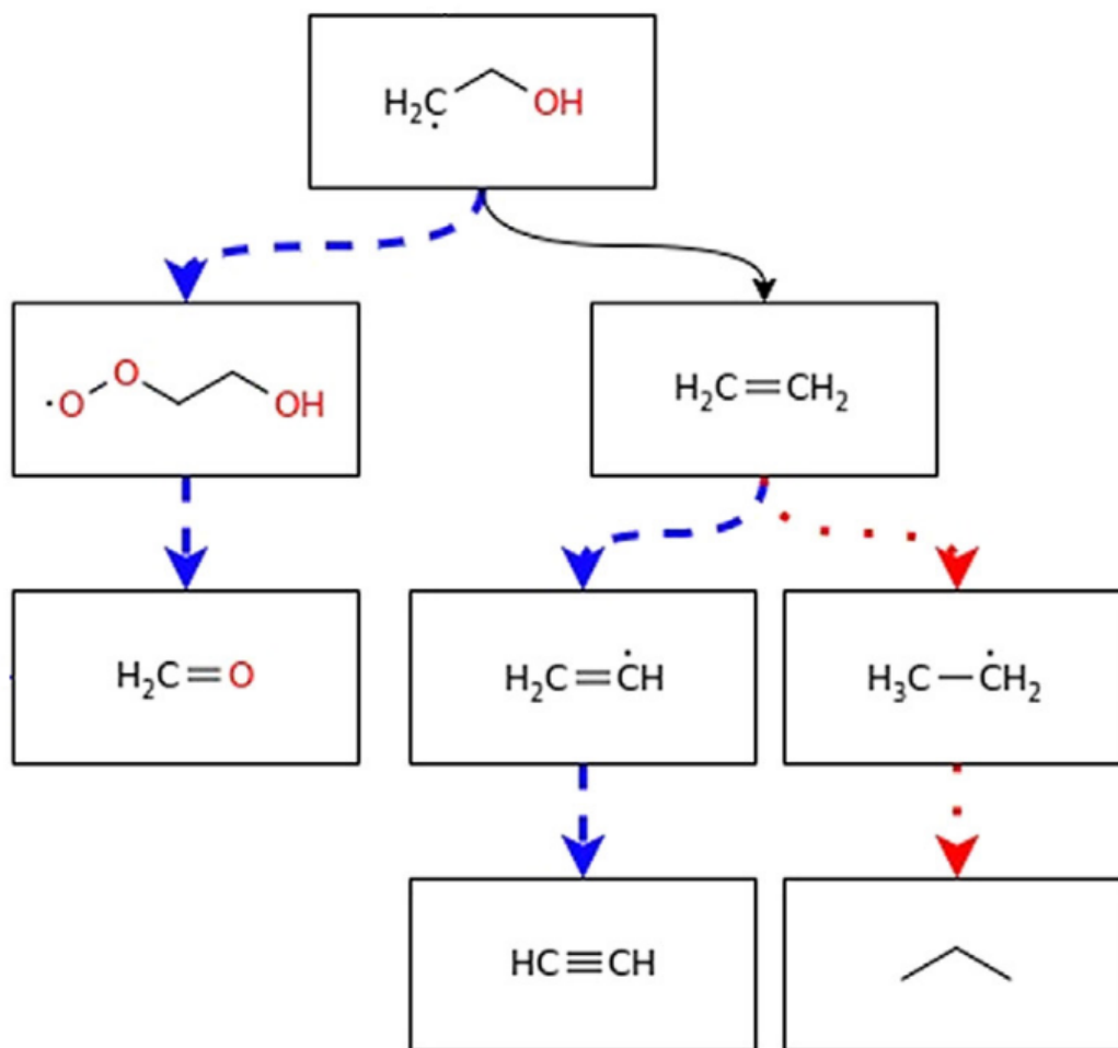
Figura 2.7: Consumo do 2-hidroxi-etil durante a RVOE na forma de estruturas moleculares. Fonte: (PIO et al., 2021).
