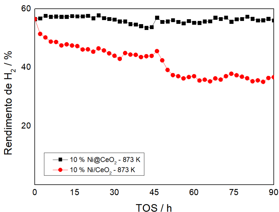
Figura 4.28: Rendimento de H_2 dos catalisadores embutidos e suportados de Ni. As reações foram conduzidas a 1 bar, 873 K por 90 h com um GHSV de 492.000 \text{ mL} \cdot \text{h}^{-1} \cdot \text{gcat}^{-1} .
