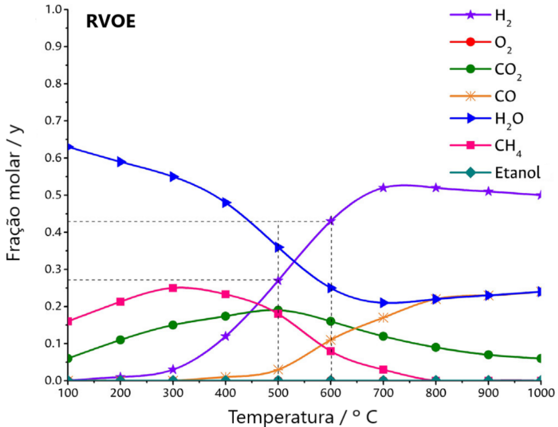
Figura 2.2: Variação dos produtos da reforma a vapor oxidativa de etanol usando uma razão \text{H}_2\text{O}/\text{EtOH}/\text{O}_2 de 3:1:0.5, com ausência de catalisador em um reator Gibbs. Adaptado de: (RODRÍGUEZ et al. , 2023).
