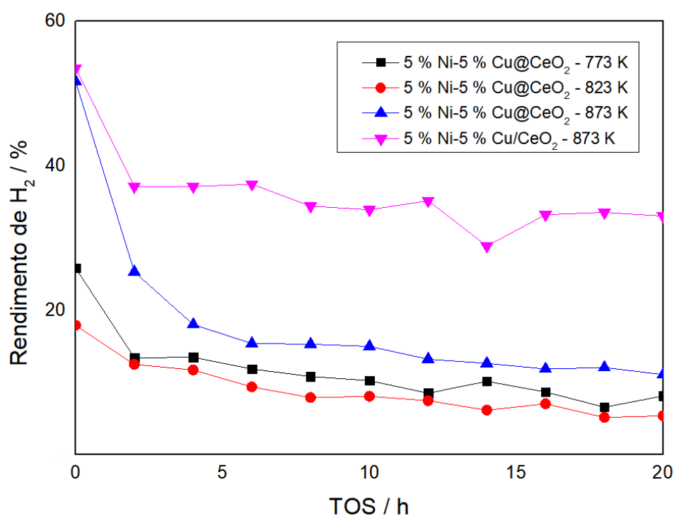
Figura 4.23: Rendimento de H_2 dos catalisadores embutidos e suportados de Ni-Cu. As reações foram conduzidas em 1 bar, a 773 K, 823 K e 873 K por 20 h com um GHSV de 492.000 \text{ mL} \cdot \text{h}^{-1} \cdot \text{gcat}^{-1} .
